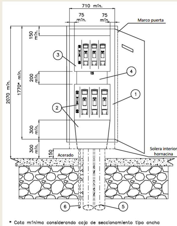
Instalación CGP y CS montaje vertical. Alzado.
