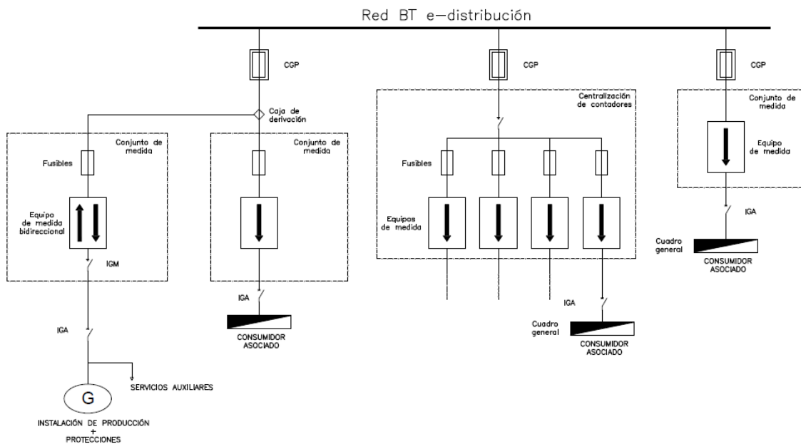
Esquema 17: Autoconsumo colectivo con excedentes (Conexión en derivación individual o en línea general de alimentación)
