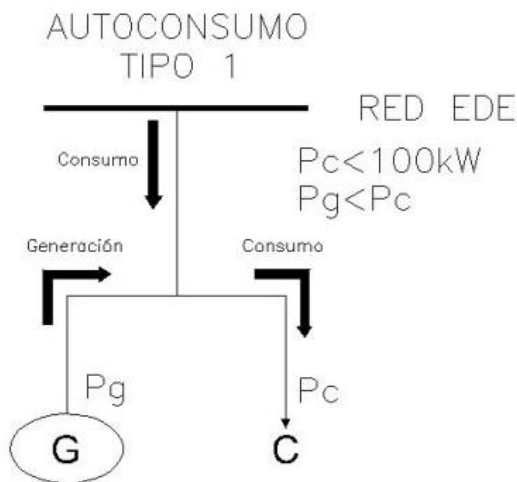
Figura 1. Autoconsumo tipo 1
