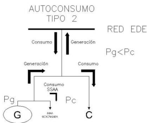
Figura 2. Autoconsumo tipo 2
